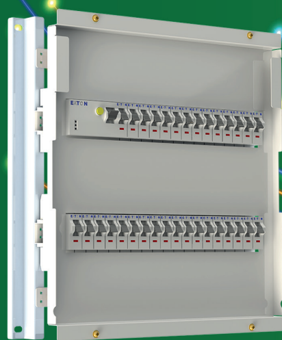
CHASSI COM ESPELHO DE PROTEÇÃO - IP 2X (03 ETAPA) TESTES E CONFIRMAÇÃO DOS CIRCUITOS
