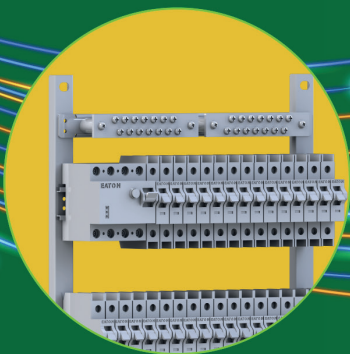
BARARRAMENTO NEUTRO ISOL. EPOX / TERRA
